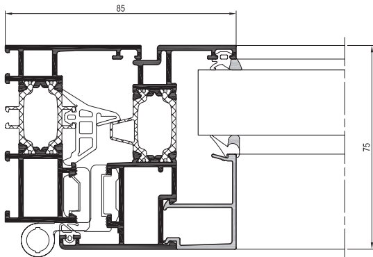
Sezione orizzontale
